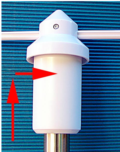
5. Poussez la base vers le haut et bloquez-la en la tournant vers la droite.
